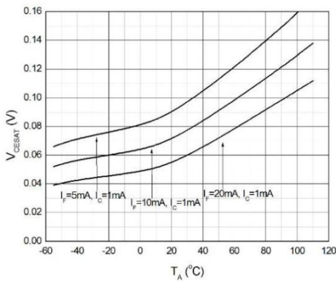
图例 9-集电极-发射极饱和压降与环境温度曲线图
